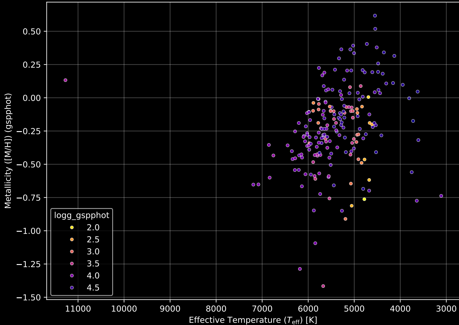
APOGEE DR17 Field: [163+78_MGA] Stellar Population Parameters (n= 207)
